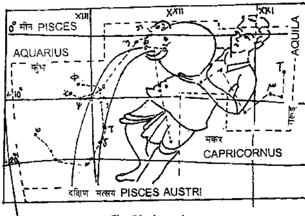
Fig. 20 Aquarius
