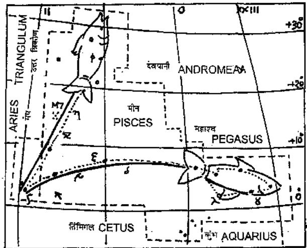
Fig. 21 Pisces
