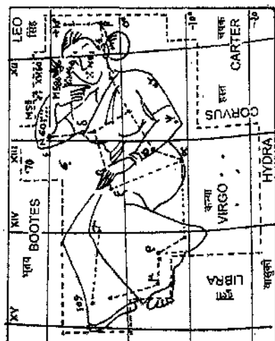
Fig. 15 Virgo
