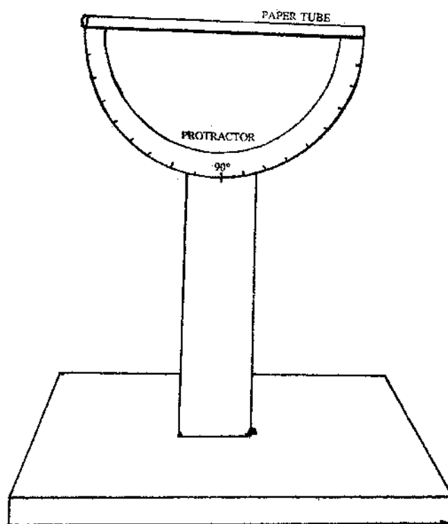
Fig. 68 Altitude Meter
