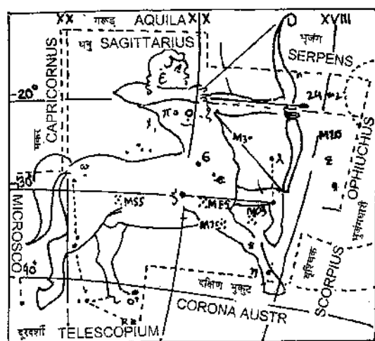
Fig. 18 Sagittarius
