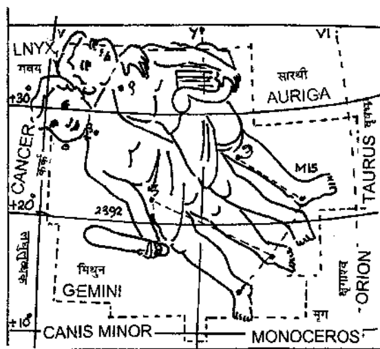
Fig. 12 Gemini
