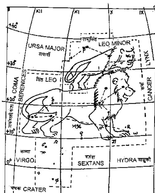
Fig. 14 Leo
