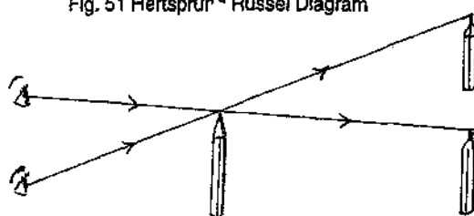
PARALLAX Fig. 52
