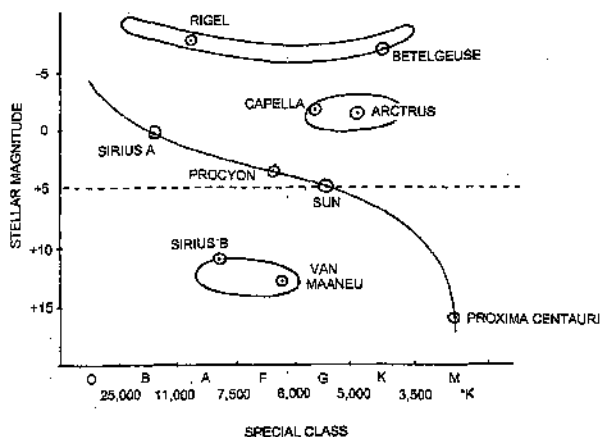
Fig. 51 Hertzsprung - Russel Diagram
